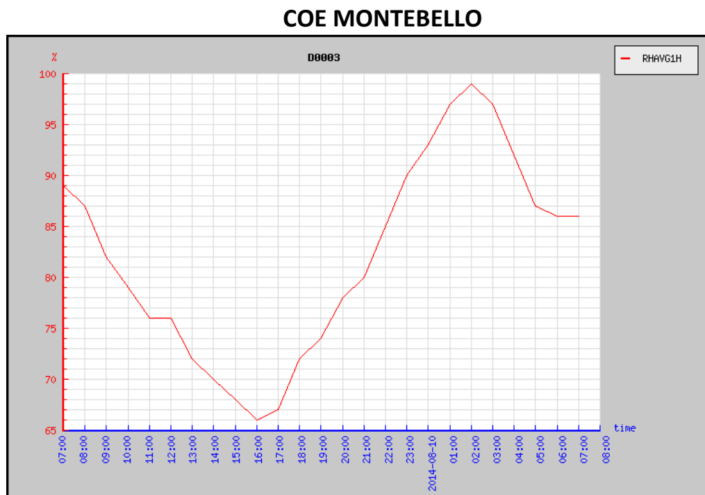
Gráfico: Humedad Relativa Promedio de 1 hora (RHAVG1H) (%)
