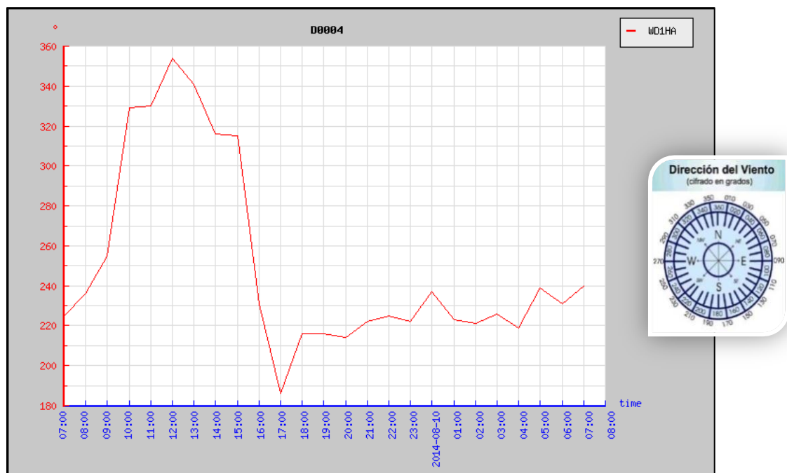
Gráfico: Dirección del viento (WD1HA) (°)
