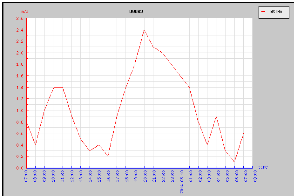
Gráfico: Velocidad del viento (WS1HA) (m/s)
