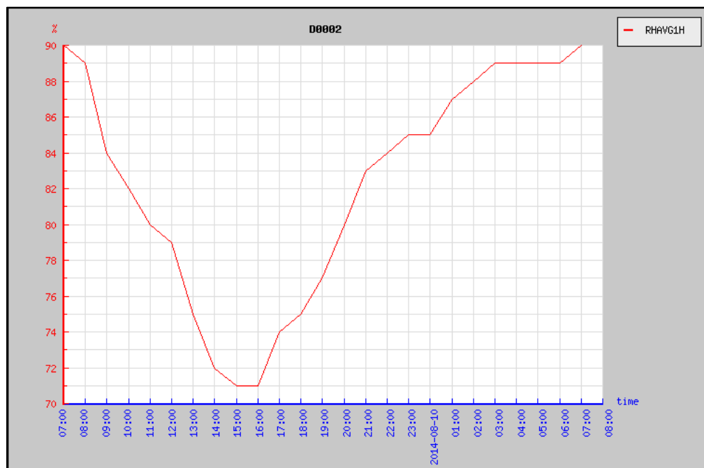
Gráfico: Humedad Relativa Promedio de 1 hora (RHAVG1H) (%)
