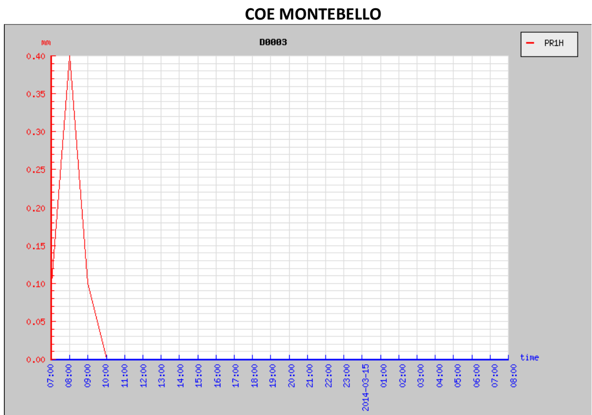
Gráfico: Precipitación acumulada (PR1H) (mm)
