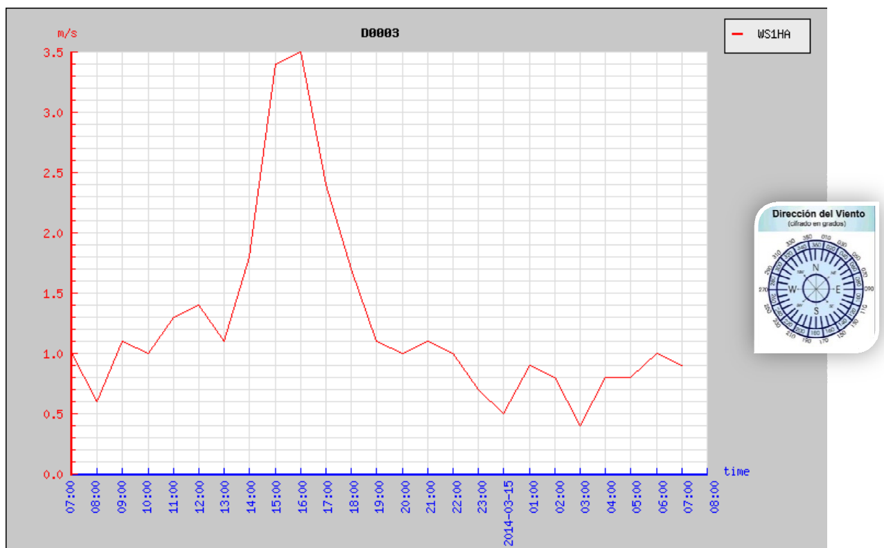
Gráfico: Velocidad del viento (WS1HA) (m/s)
