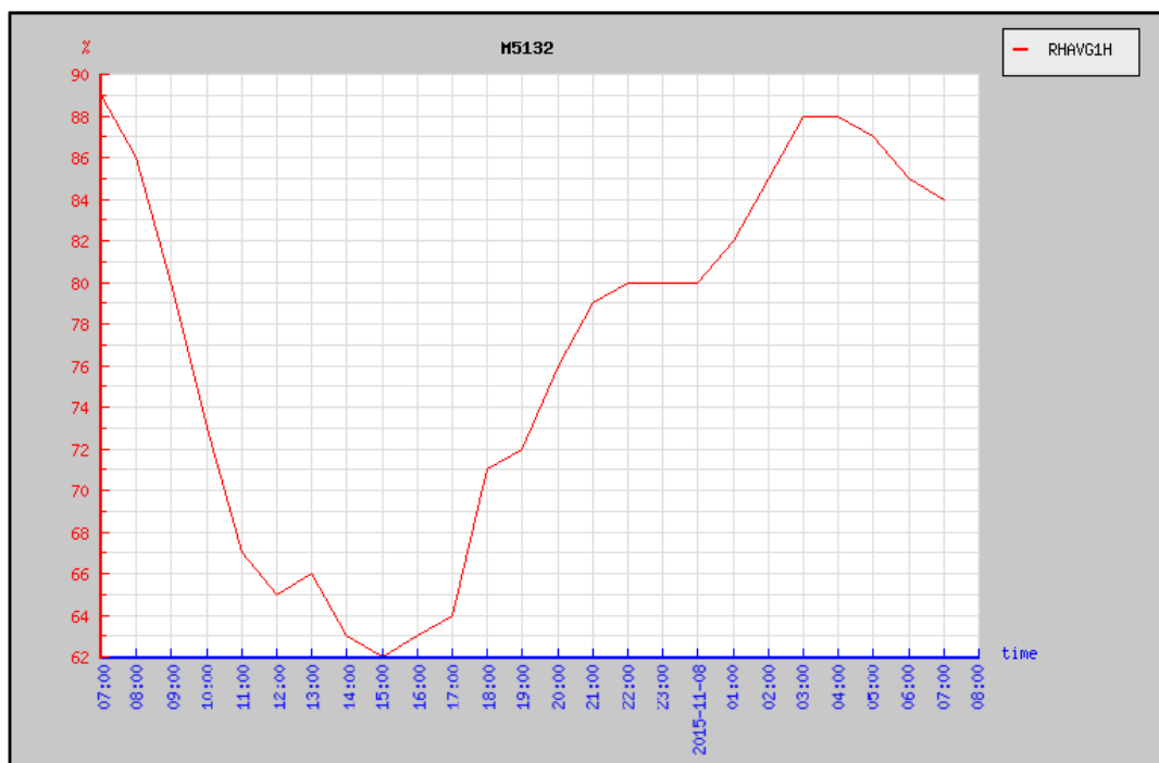
Gráfico: Humedad Relativa Promedio (RHAVG1H) (%).
