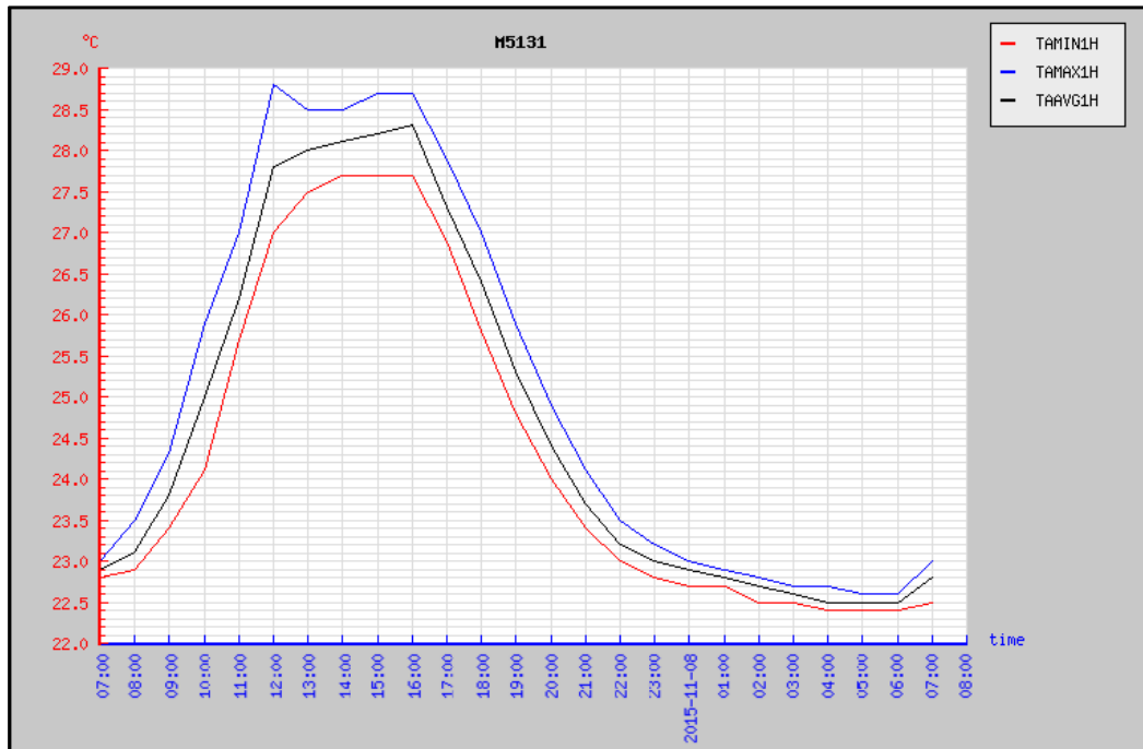
Gráfico: Temperatura Promedio, Máxima y Mínima (°C)
