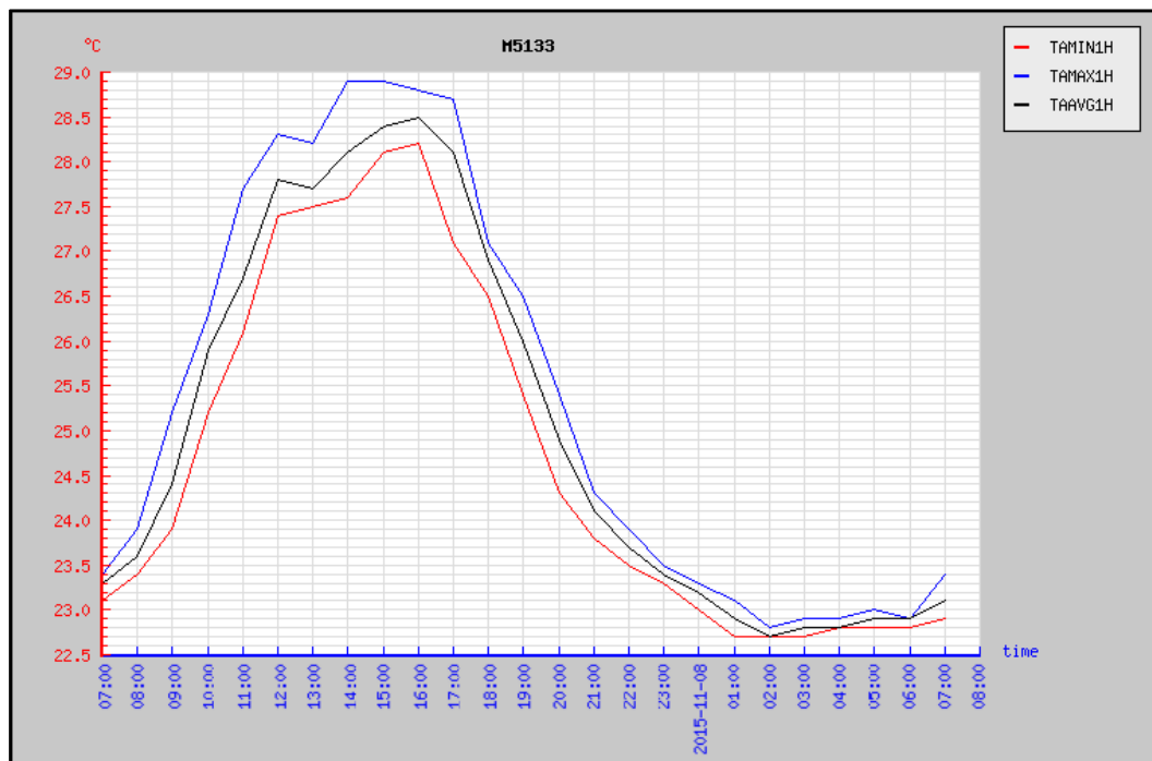
Gráfico: Temperatura Promedio, Máxima y Mínima (°C).
