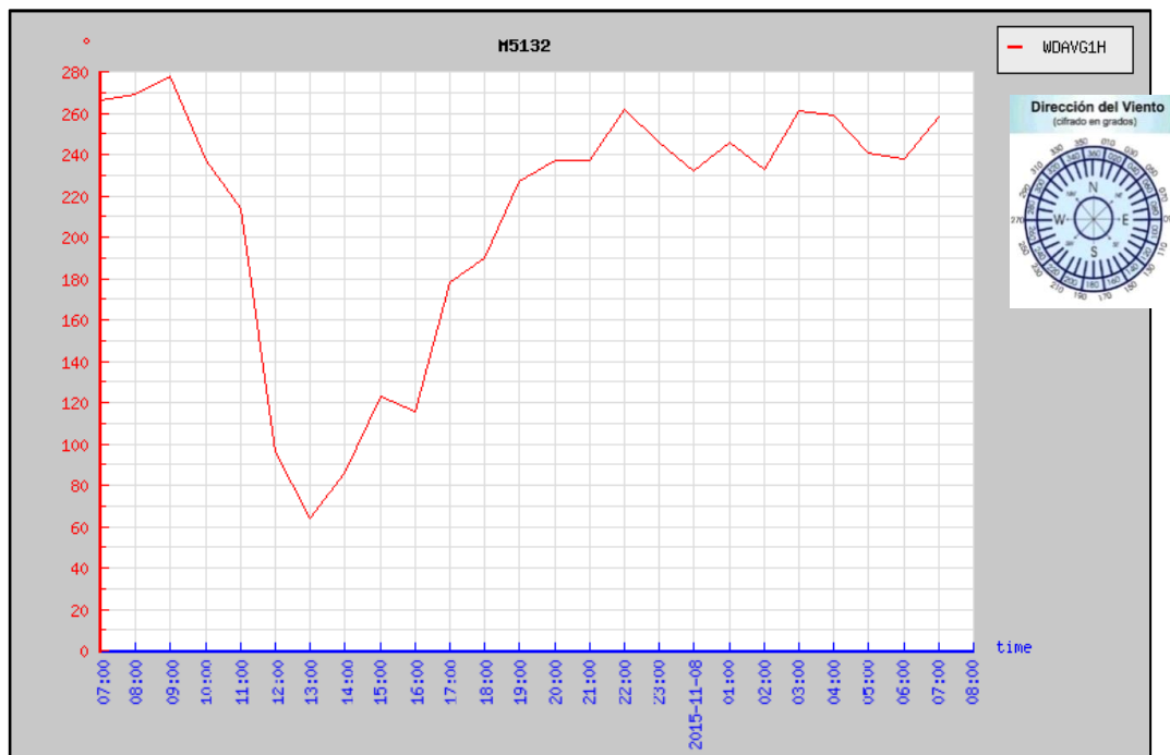
Gráfico: Dirección del Viento Promedio (WDAVG1H) (°).
