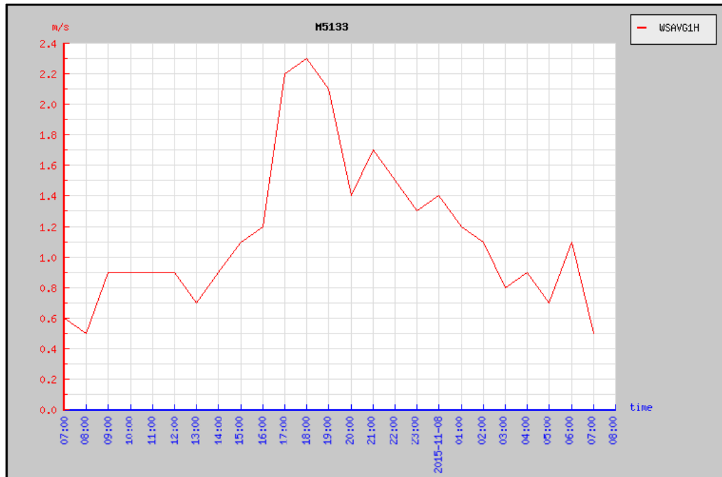
Gráfico: Velocidad del Viento Promedio (WSAVG1H) (m/s).
