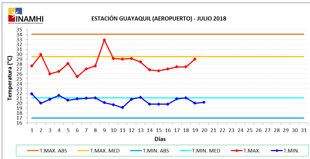
Figura 1: Registro diario de temperaturas extremas durante el mes de julio de 2018 en Guayaquil, tomando como referencia la estación Aeropuerto (DAC).
