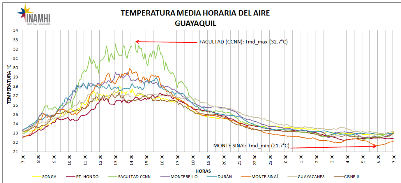
Figura 4: Temperatura media del aire registrada en las Estaciones Meteorológicas Automáticas desde las 07h00 del miércoles 26 de mayo hasta las 07h00 del jueves 27 de mayo de 2021.
