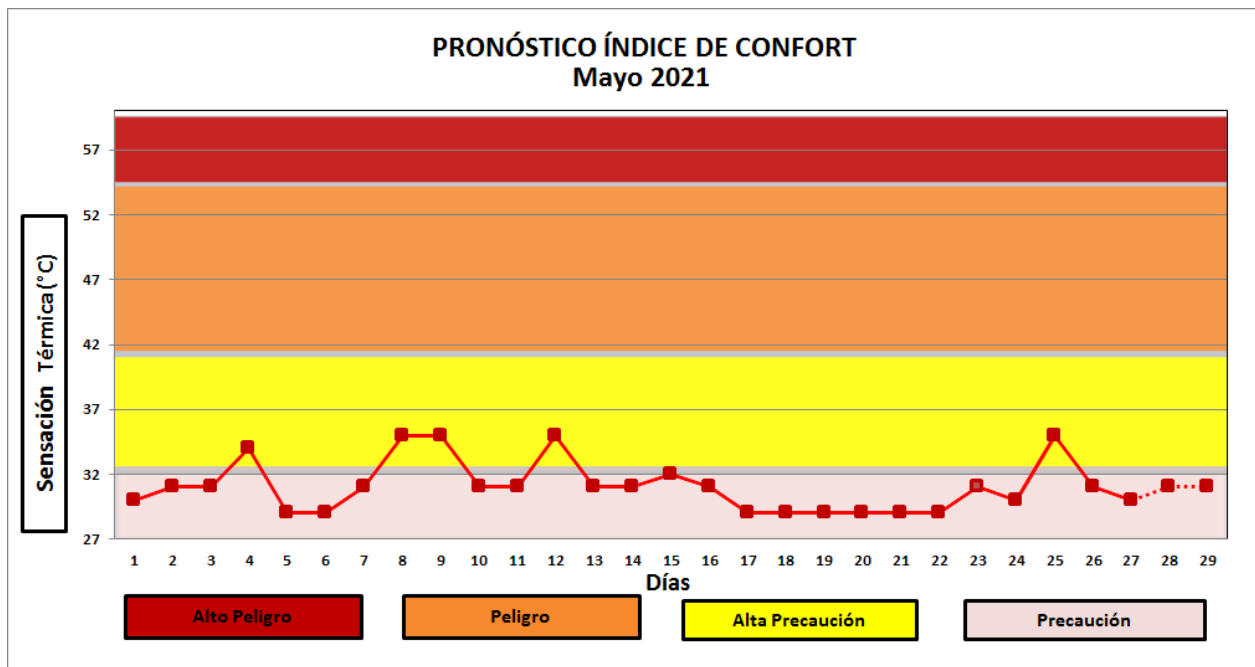
Figura 6: Índice de Confort: la línea continua se corresponde con los valores reales tomando como referencia la estación EMA Facultad CCNN (UG). La línea punteada indica el valor pronosticado para el día 28 y 29 de mayo de 2021.
