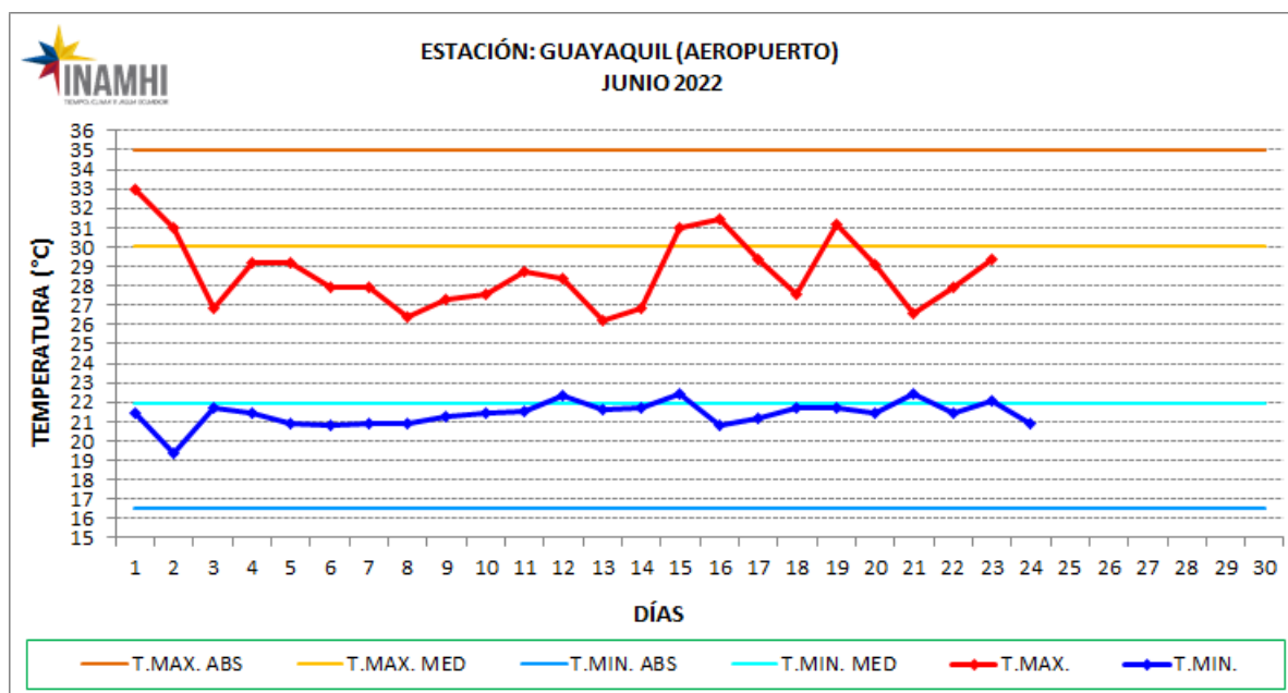
Figura 4: Registro diario de temperaturas extremas durante el mes de junio del 2022 en Guayaquil tomando como referencia la Estación Guayaquil Aeropuerto - DAC.
