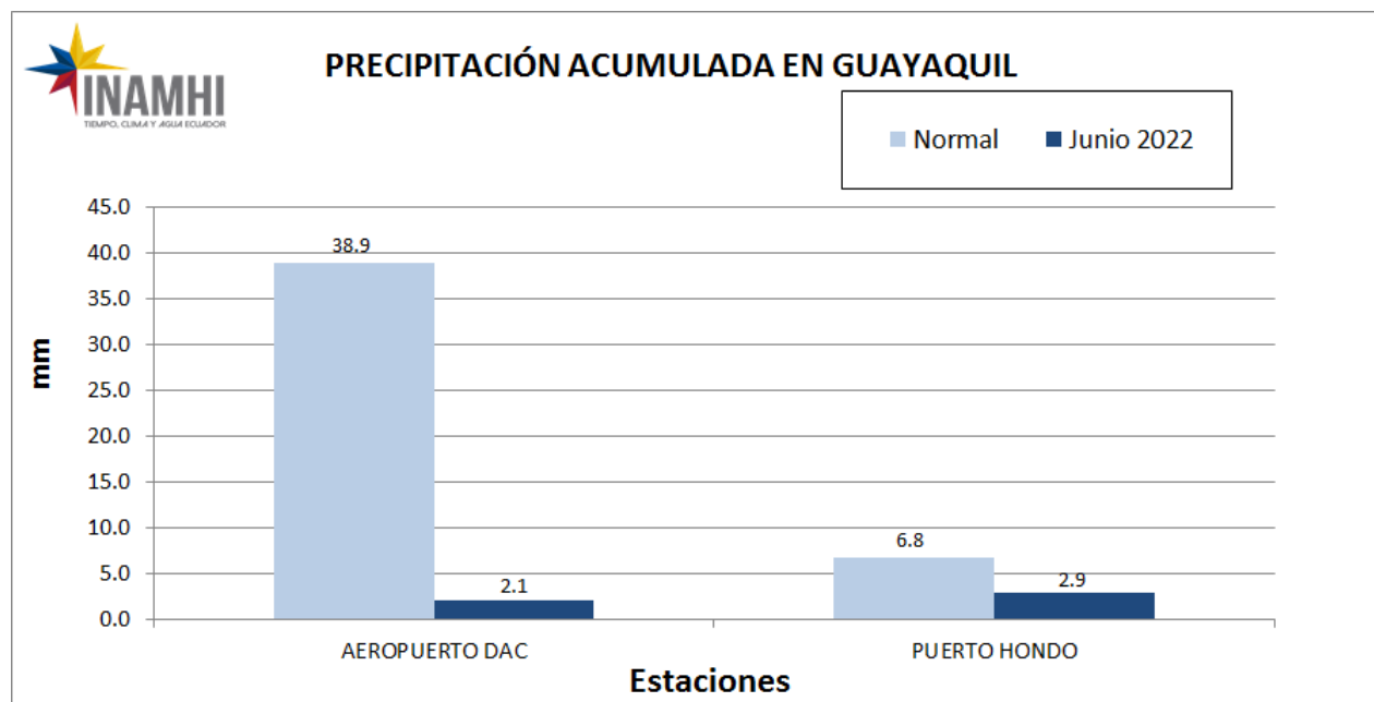
Figura 1: Lluvia acumulada durante el mes de junio de 2022 en Guayaquil, tomando como referencia las estaciones Aeropuerto (DAC) y Puerto Hondo.
