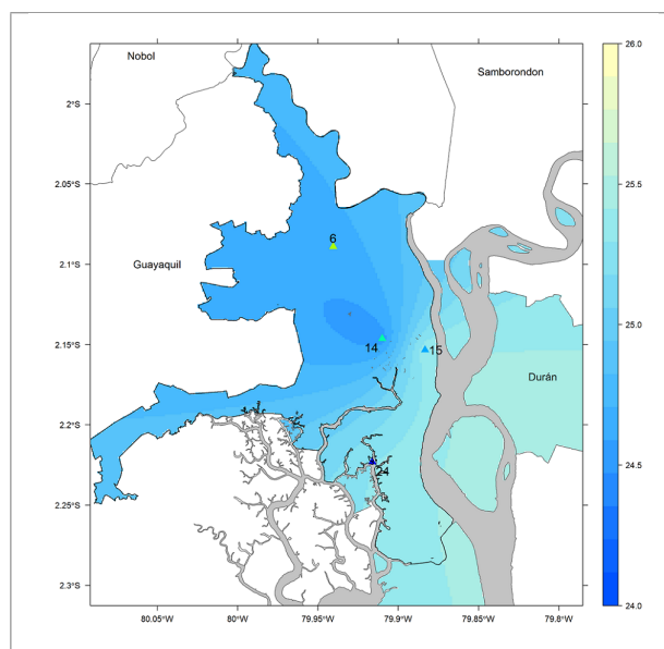
(b) Temperatura mínima promedio Mayo 2023
