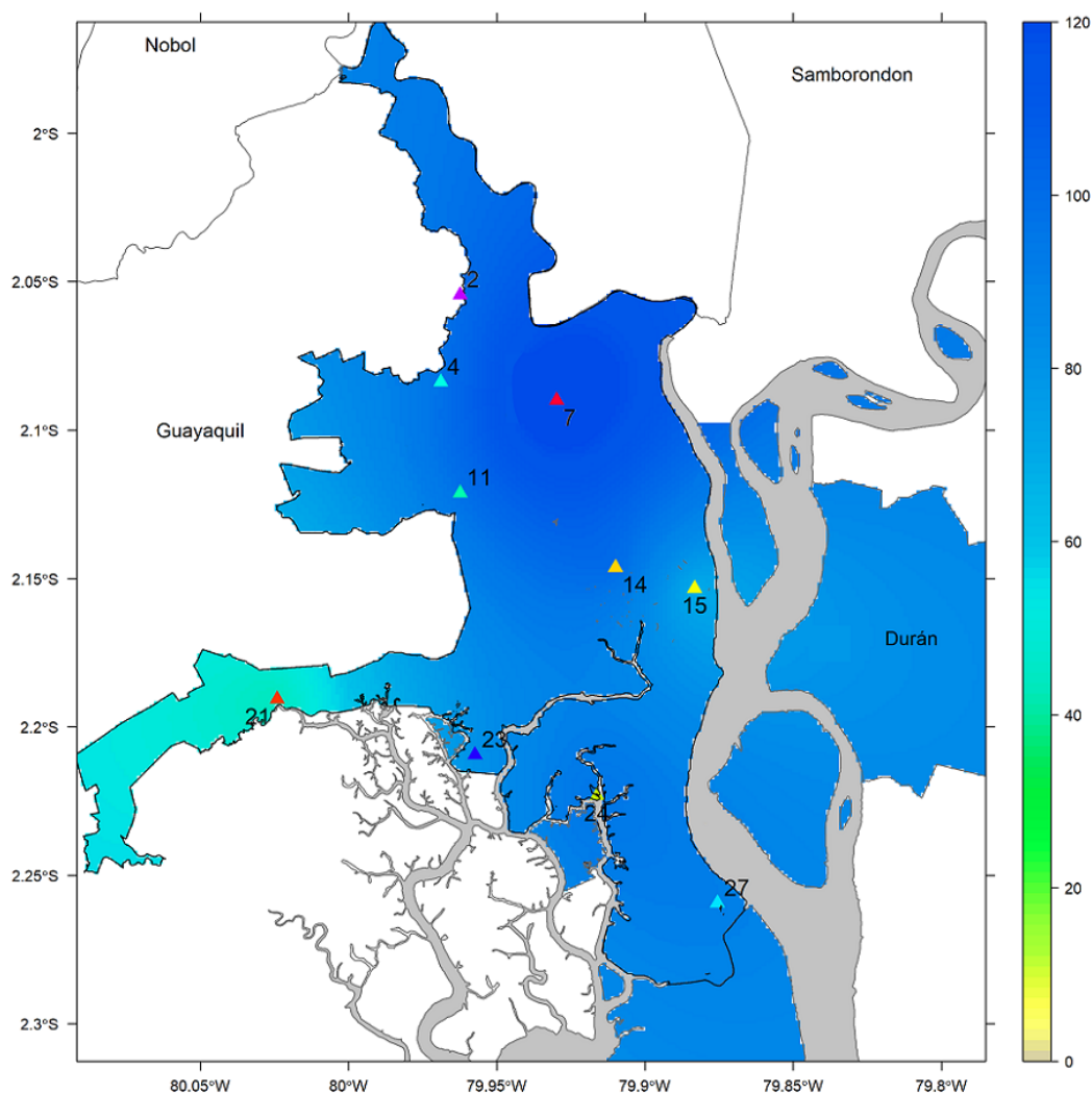
Figura.1 Mapa de precipitación Guayaquil- Mayo 2023.
