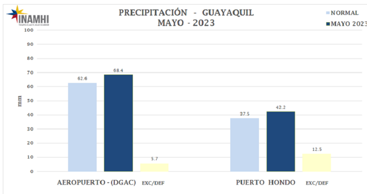
Figura 2: Precipitación Mayo 2023 Guayaquil: Aeropuerto (DGAC), (PV) Puerto Hondo.
