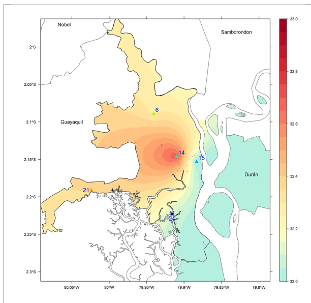
(a) Temperatura máxima promedio, Mayo 2023
